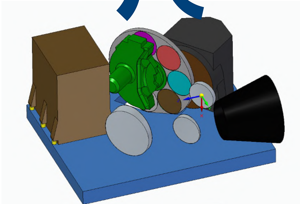
RUEDAS DE FILTROS JUICE-JANUS
